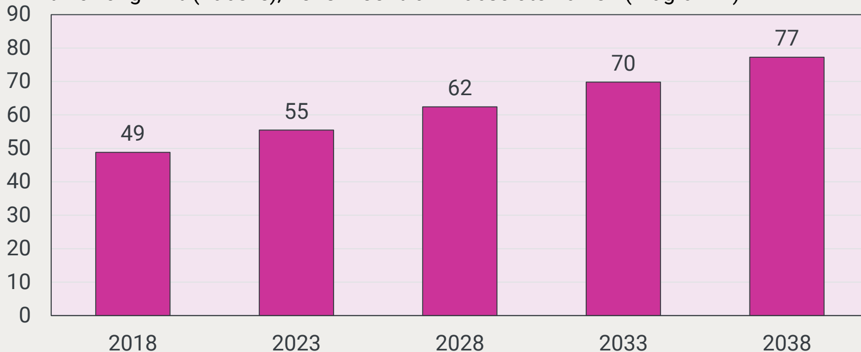
Entwicklung in % (Tabelle), 2018=100 % bzw. absolute Zahlen (Diagramm)
