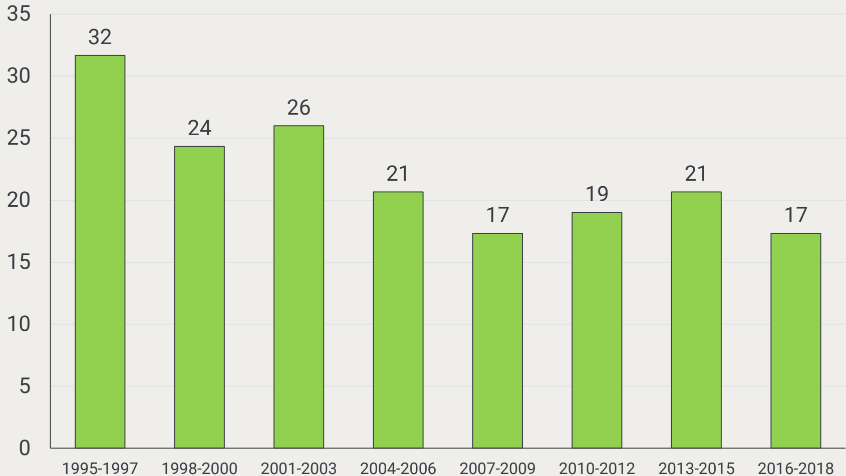
Entwicklung der Geburtenzahlen 1995 - 2018
