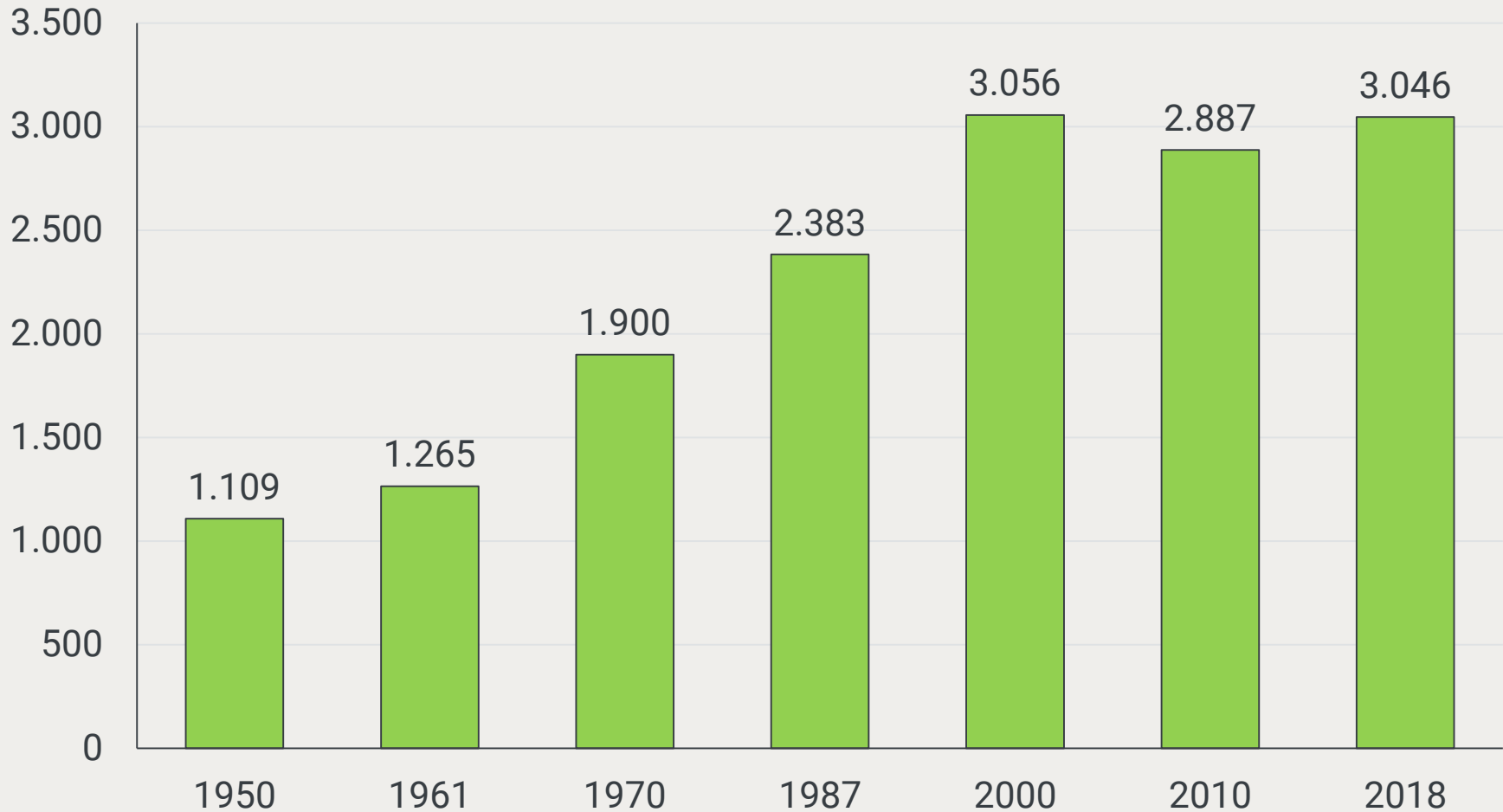
Entwicklung der Einwohnerzahlen 1950 - 2018
