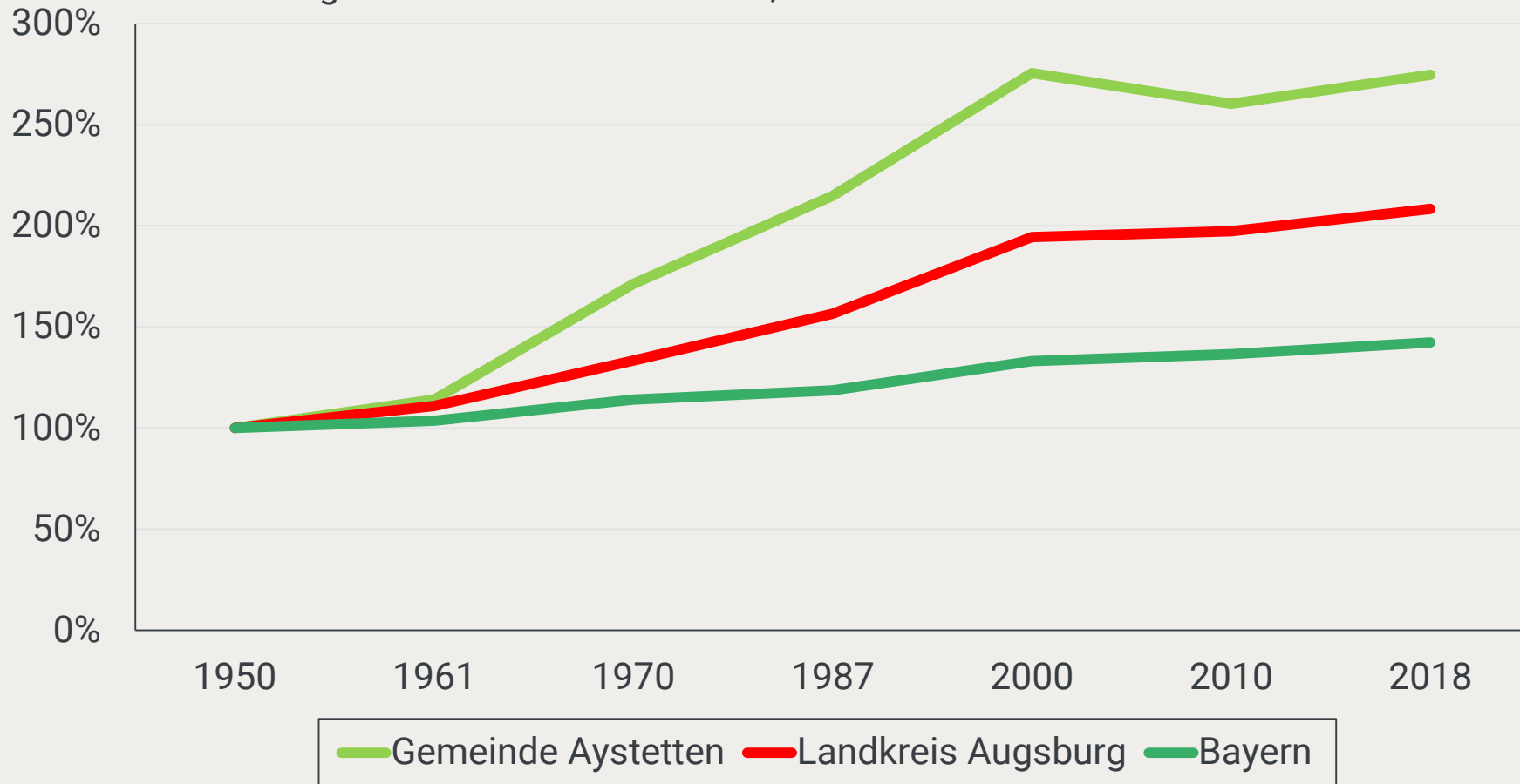
Entwicklung der Einwohnerzahlen in %, 1950=100 %
